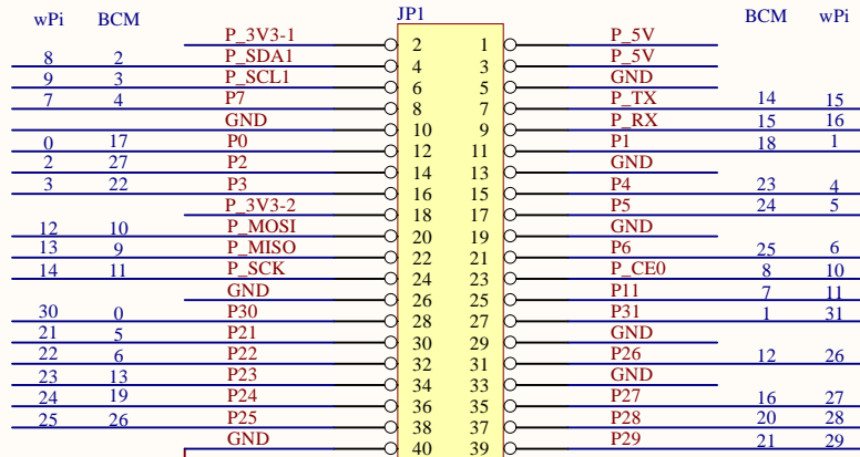
双排插装排母2*20 40PIN 2.54间距
